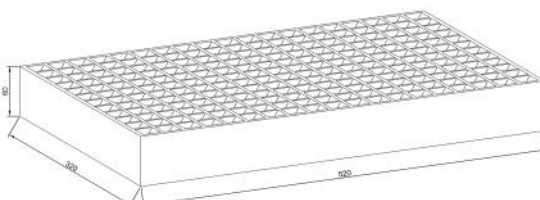
SEMILLERO 228 CAVIDADES
