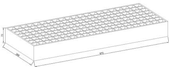
SEMILLERO 168 CAVIDADES
