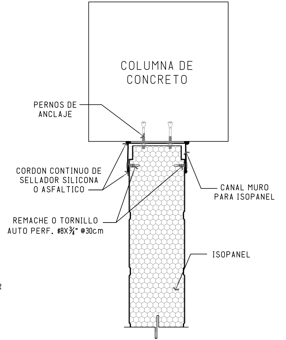
DETALLE DE UNION ISOPANEL - COLUMNA
