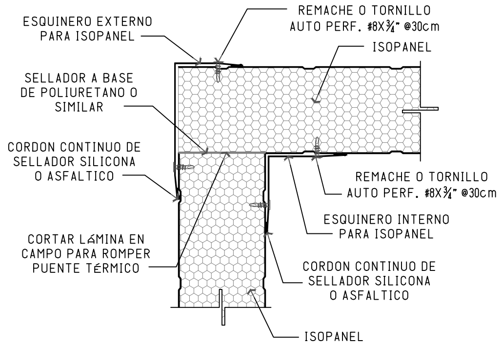
DETALLE DE UNION EN ESQUINAS
