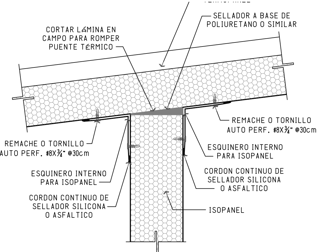
DETALLE DE UNION DE ISOPANEL CON CUBIERTA DE TERMOPANEL
