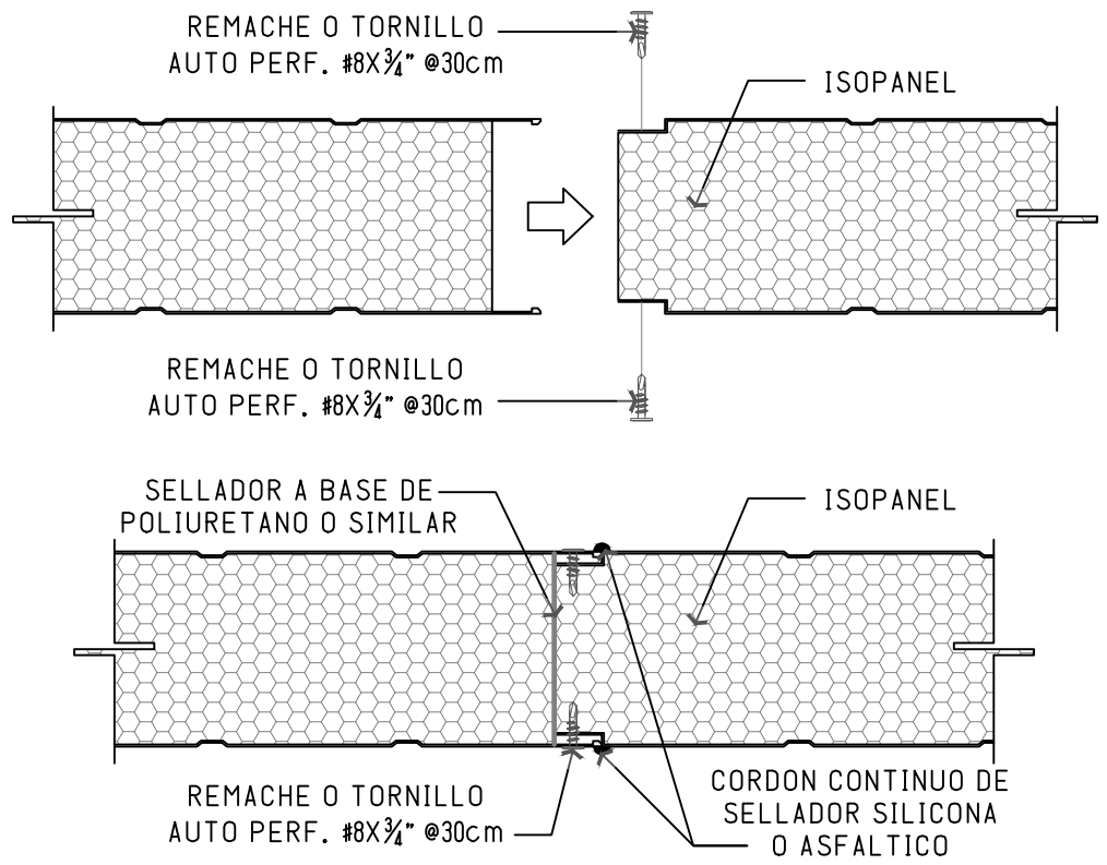
DETALLE DE UNION DE ISOPANELES
