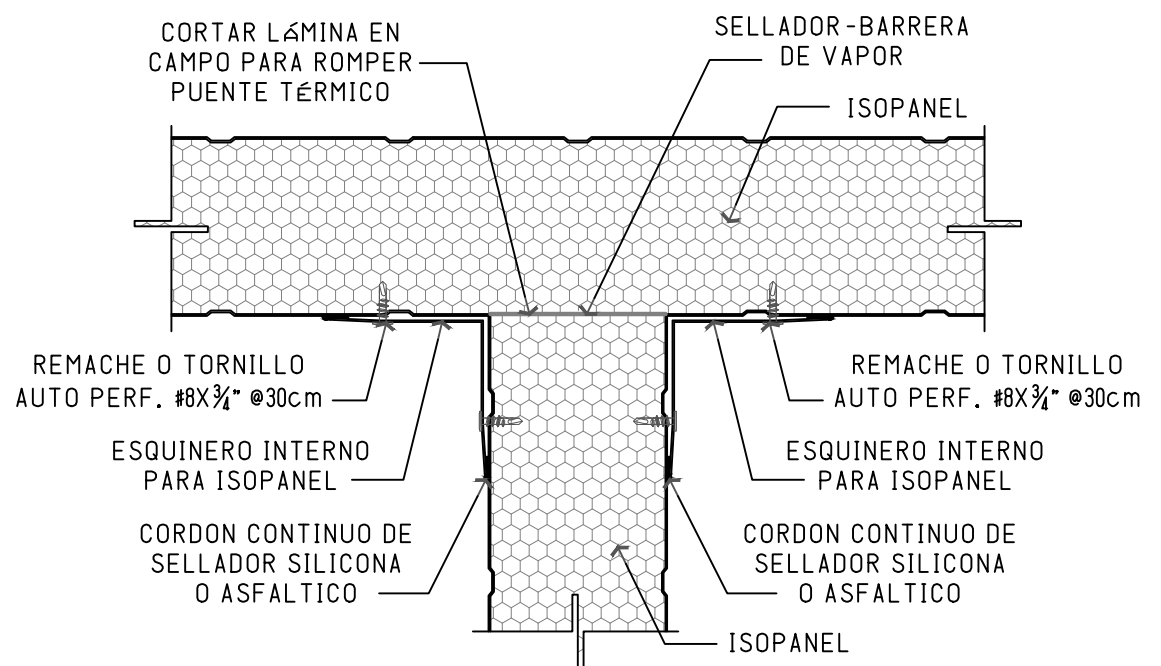
DETALLE DE UNION EN "TEE"
