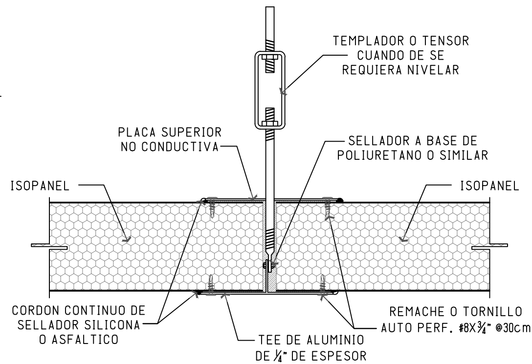
1 ALTERNATIVA DE CIELO SUSPENDIDO CON ISOPANEL
