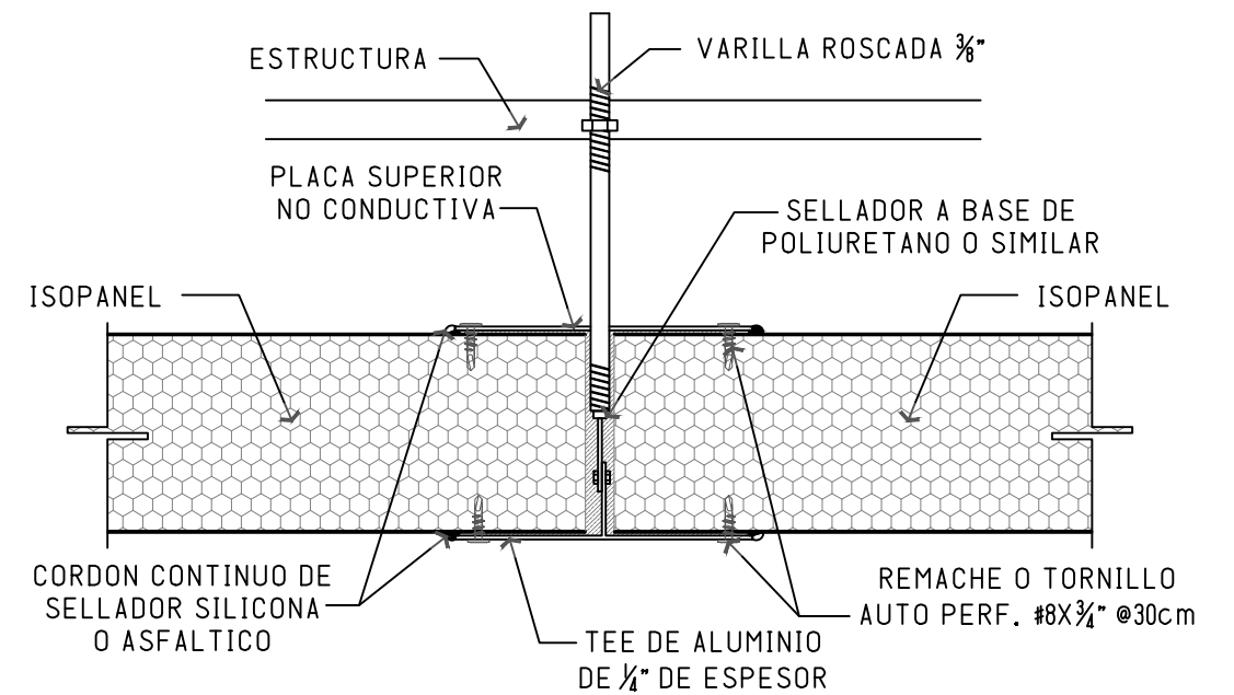
2 ALTERNATIVA DE CIELO SUSPENDIDO CON ISOPANEL
