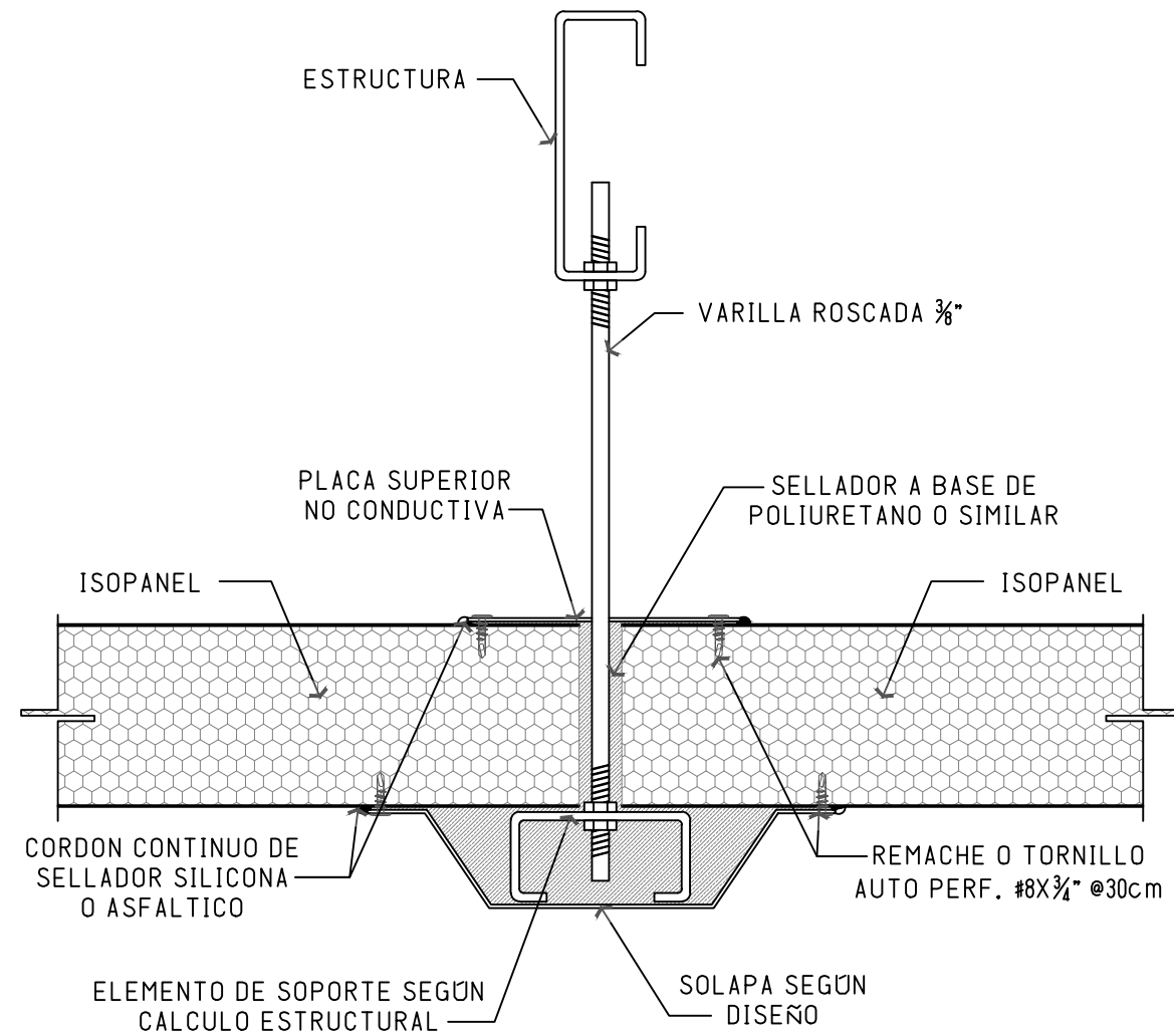
1 ALTERNATIVA DE CIELO SUSPENDIDO CON ISOPANEL
